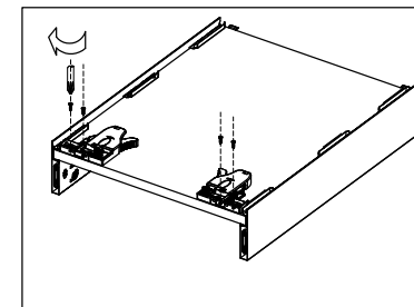
Монтаж фиксаторов
