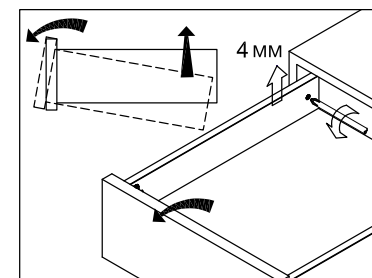
Регулировка наклона
