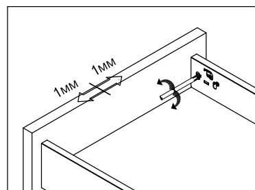
Горизонтальная регулировка
